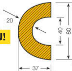
BOGEN 60
